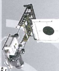
Scheibentransportanlage 25/50/100 m Als Match und Turnier
