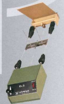
Scheibenzuganlage 10 m
